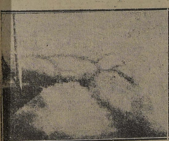
MAZ DE NUBES FOTOGRAFIADO DESDE UN AVION CUMULUS-STRATUS
