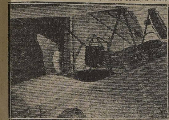
DISPOSICIONES DE LOS INSTRUMENTOS METEOROLOGICOS EN UN AVION DESTINADO A INVESTIGACIONES AEREOLOGICAS
