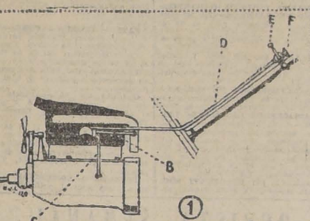
FIG. 1. — Montaje del economizador. — B, derivación del escape; C, toma del gas del carter; D, conducto de aire fresco; E, llave de paso; F, embudo.
