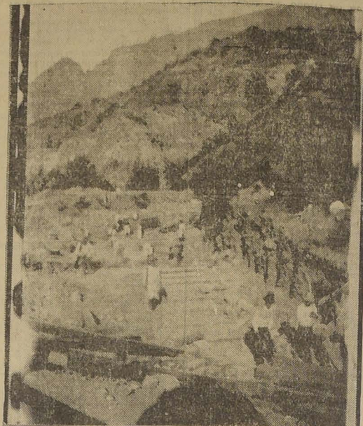
COLOCANDO EN LAS INMEDIACIONES DEL TUNEL N.º 3, LOS SOPORTES DE MADERA CON QUE SE ESTAN HACIENDO LAS REPARACIONES
