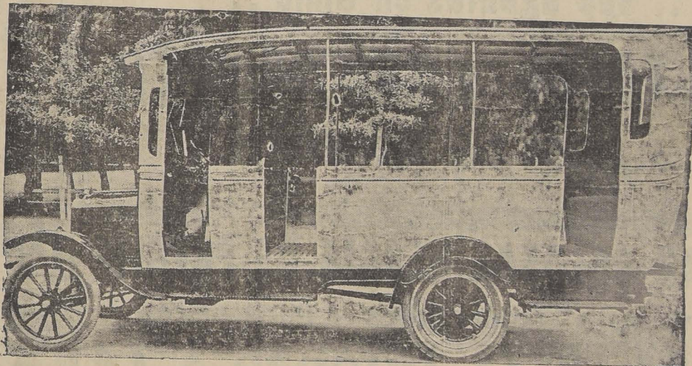
MODELO STANDARD DE CARROCERIA PARA FORD
