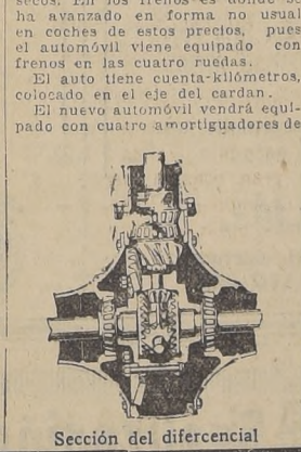
Sección del diferencial
