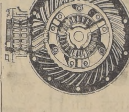
Engranaje espiral de la corona
