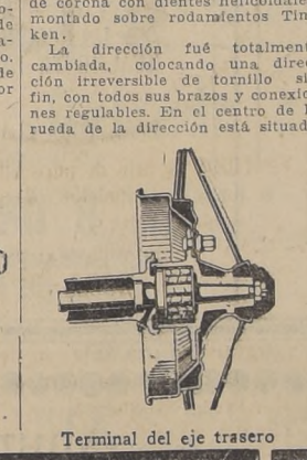
Terminal del eje trasero
