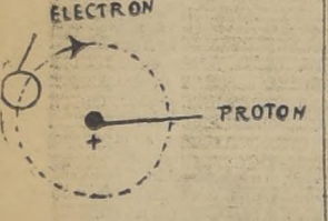
Atomo de hidrógeno, según Bohr.
