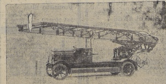
La telescópica "Magirus" después de armada
