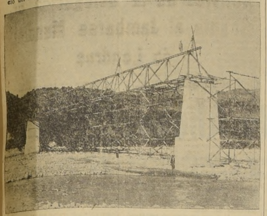
Estado del puente sobre el Cachoapoal para el paso de la cañería del agua potable, el 26 de II-1929
