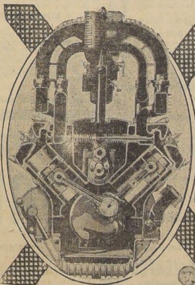
Sección del nuevo motor V de ocho cilindros, que demuestra la acción de la válvula horizontal única.
