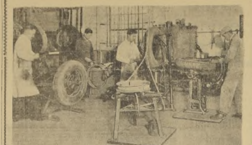
Los aparatos Weaver se usan en todas las somerías del mundo. La gomería que aparece en el grabado superior emplea las cámaras neumáticas Weaver. El Modelo E a mano y el accionado a aire comprimido para desmontar los neumáticos de las llantas seccionadas; el extractor automático de neumáticos a aire comprimido; el Sacallantas Weaver para desmontar los neumáticos pesados usados en omnibuses y camiones y el yunque para llantas.
