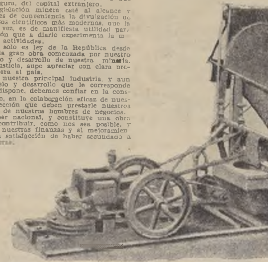
Maquina separadora de oro, por el sistema cen trifugo. Esta pequeña máquina, de un peso aproximado de 350 kilos, ha dado, en Estados Unidos, excelentes resultados. Se ayuda de un motorcito a gasolina, de económico gasto, y lava a, en ocho horas de trabajo, poco más de cincuenta toneladas.
