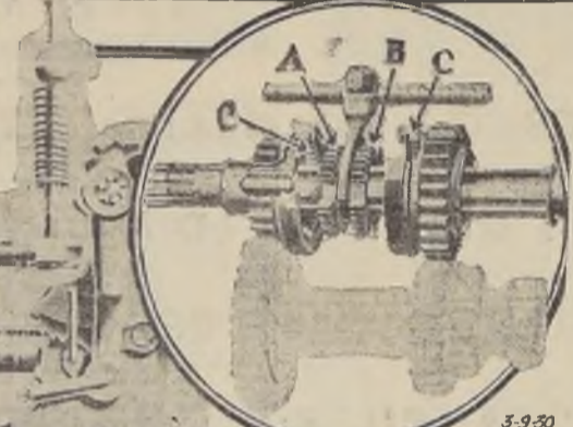
3.—ENGRANAJES INTERNOS DE TRANSMISION, MARCADOS CON LA LETRA C, Y LOS EXTERNOS SIGNADOS CON LA LETRA A.
