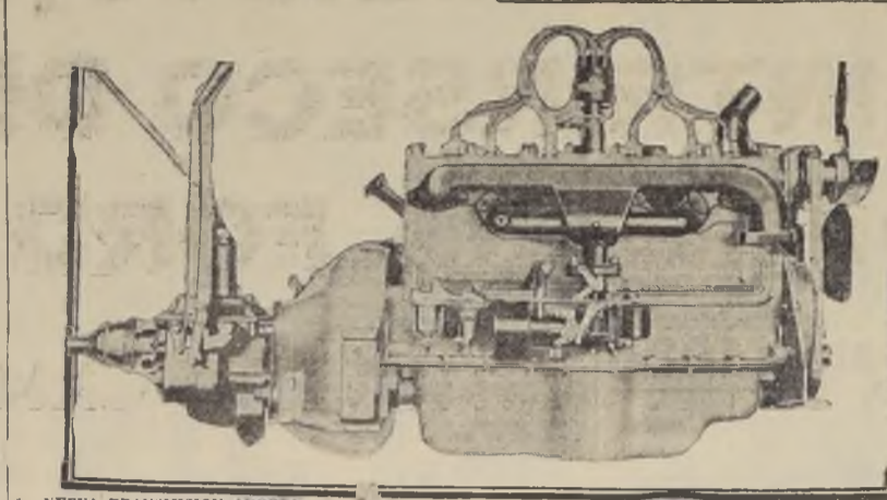
1.—NUEVA TRANSMISION ADOPTADA POR UN DESTACADO FABRICANTE EN LOS ULTIMOS MESES, EMPLEANDO ENGRANAJES DE "ESPINA DE ARENQUE".
