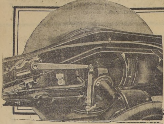
EL FRENO Y EL AMORTIGUADOR COLOCADO EN EL CHASSIS. NOTENSE LOS COJINETES Y DEMAS PARTES DONDE LA LUBRIFICACION ES NECESARIA.
