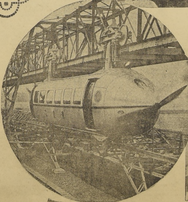
Esta vista del railplano muestra cómo el vehículo está suspendido de los rielos. Nada descansa en la estructura situada debajo de él, la cual solamente existe para el contrabalanceo del aparato.
