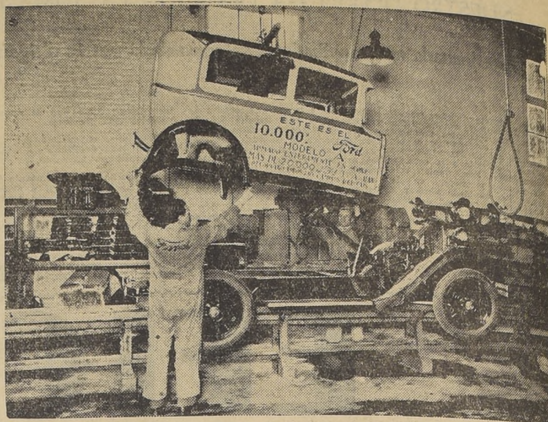
En la línea de montaje de la Sucursal de Santiago de la Ford Motor Company. Se ve en el momento de montar la carrocería modelo Tudor en el 10.000.º Ford modelo "A" enteramente armado y acabado en Chile.
