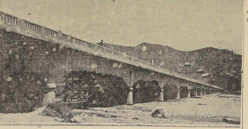
El puente sobre el río Aconcagua, que será inaugurado el sábado próximo. Tiene dos calzadas.
