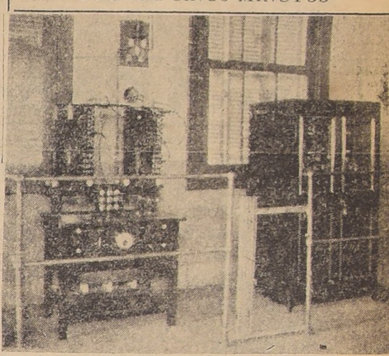
Los aparatos transmisores de la radio-estación de "El Bosque".
