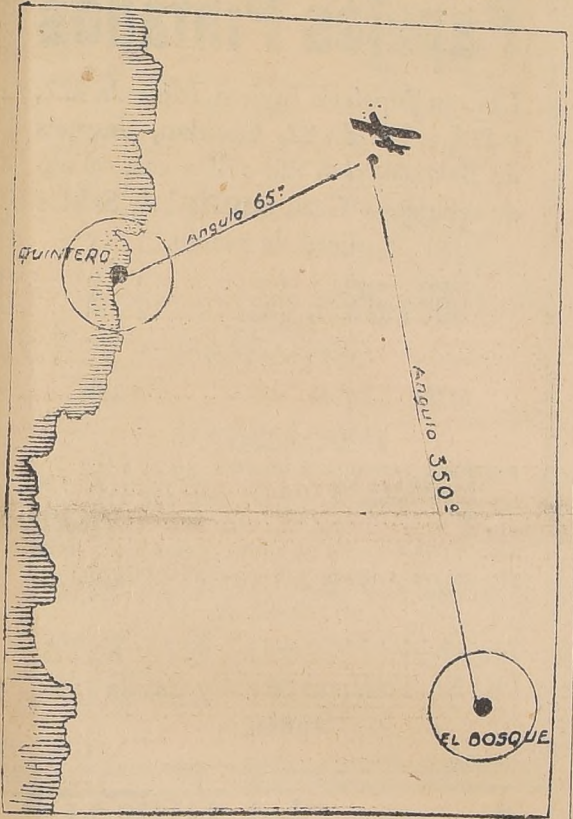
Como se indica la posición geográfica de un avión en vuelo.
