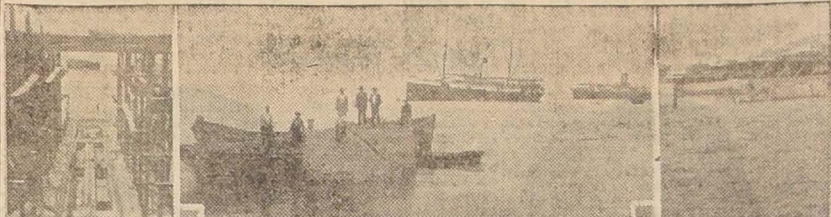
De izquierda a derecha: 1. Uno de los varaderos.—2. El fondeamiento del primer cajón.—3. Tres cajones fondeados. En esta forma se lo ha ganado al mar una faja de ciento sesenta y cinco metros de largo por cinco metros de ancho.
