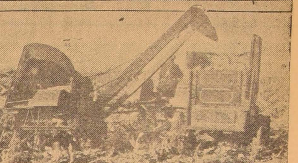
Arrancadora-deshojadora que funciona actuada por un tractor de acoplamiento directo, el cual también tira del carro cargado de espigas. Dos hombres solamente pueden recoger de 4 a 5 hectáreas de maíz por día.
