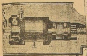
Corte transversal de un motor de arranque. Necesita una gota de aceite en cada 2,000 millas recorridas
