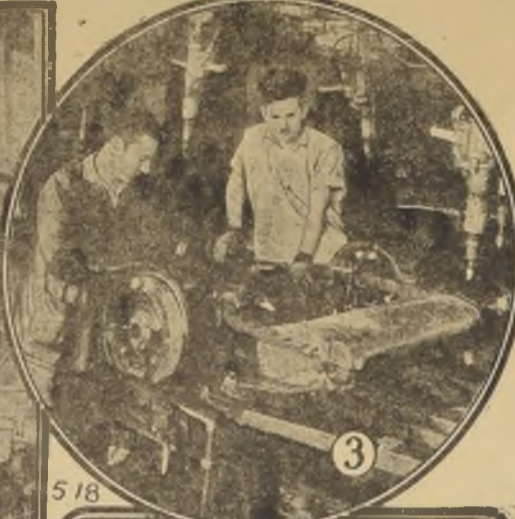
Cabecera de una de las secciones del túnel de la Ford ilustrando la maquinaria usada para horadar bajo tierra. Al frente se ve una de las planchas de concreto que se usaron para forrar el túnel. Este tiene un diámetro interior de 15 pies.
