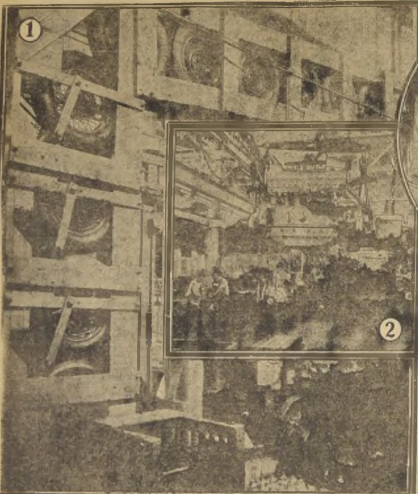
1. QUEDA TRANSMISORA QUE CONDUCE A LAS "RUEDAS" HASTA LA LINEA Y AL PUNTO NECESARIO. — 2. VISTA DE LA LINEA DE AGRUPAMIENTO DEL CHASSIS, EN UNA FABRICA DE DETROIT. LA GRUÁ DE LA PARTE SUPERIOR DEJA CAER EL ARMAZON EN EL SITIO NECESARIO. — 3. COLOCANDO LOS RESORTES Y EJES, MIENTRAS EL CHASSIS ESTA INVERTIDO. NOTESE LAS TENAZAS AUTOMATICAS QUE PENDEN DEL TROLLEY. — 4. CADA MAQUINA ES SUJETA A UNA PRUEBA ANTES DE SER COLOCADA EN EL CHASSIS.
