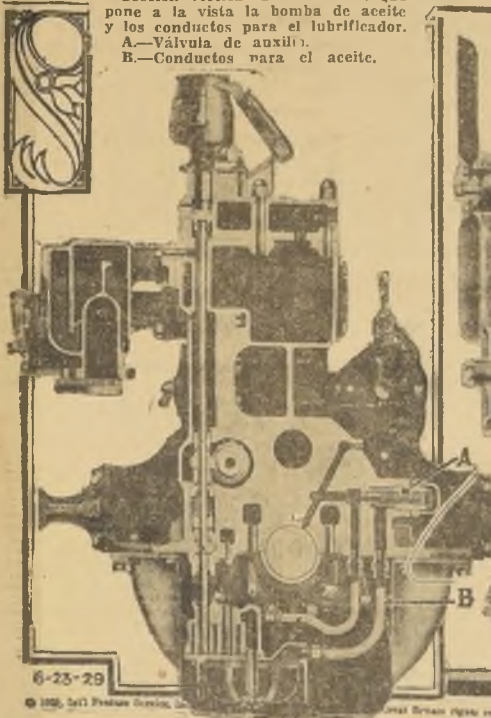
Sección de un motor de cuatro cilindros de gran desplazamiento, que indica los conductos para el aceite.
