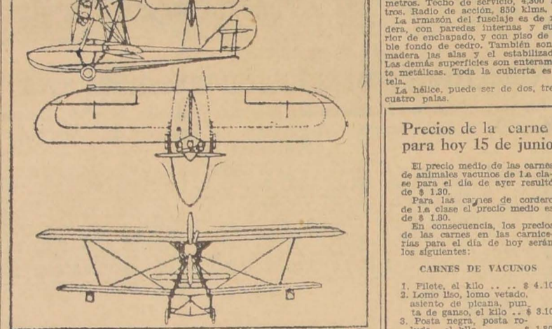
SAVOIA-MARCHETTI (Anfibio S-13). CARACTERISTICAS. — Envergadura: ala superior, 15,30 m.; ala inferior, 13,30 m. Longitud total, 10,20 m. y altura, 3,10 m. Motor Isotta-Varda...
