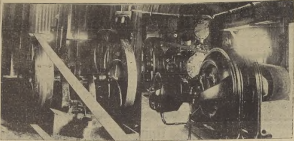
La Central de Fuerza de Andacollo, que suministra la energía a las bombas captadoras de agua y el alumbrado eléctrico a la población.
