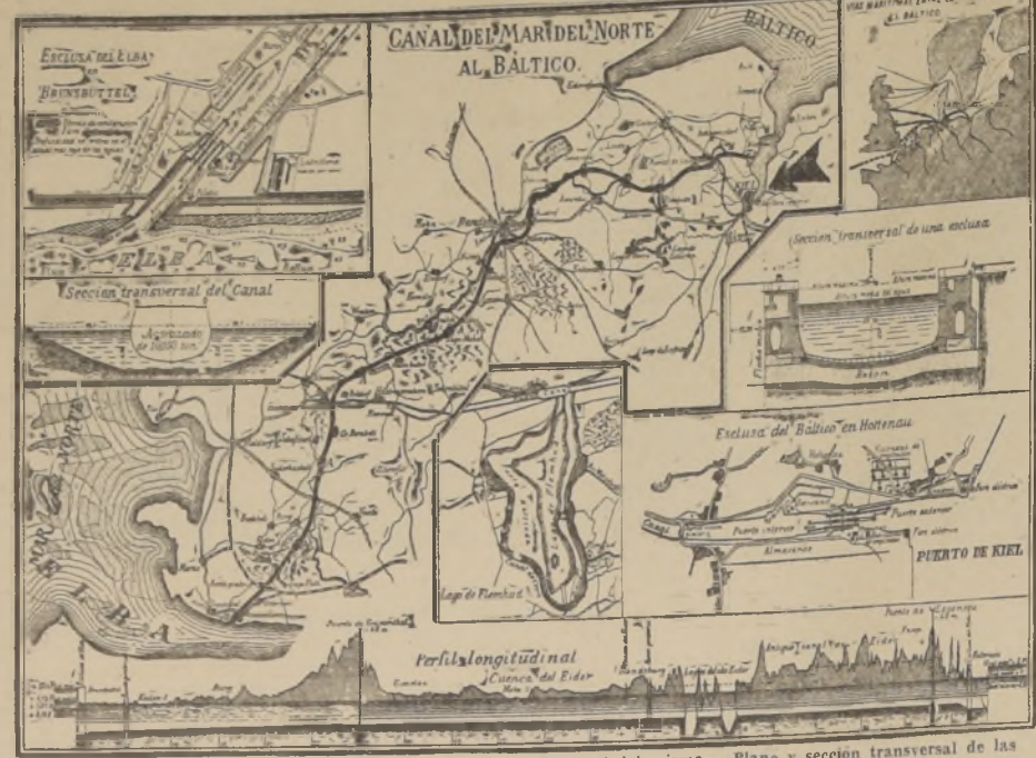
Plano del Canal de Kiel.— Perfil longitudinal y sección transversal del mismo.— Plano y sección transversal de las esclusas.— Plano del lago de Fehmuh y vias marítimas entre el mar del Norte y el Báltico
