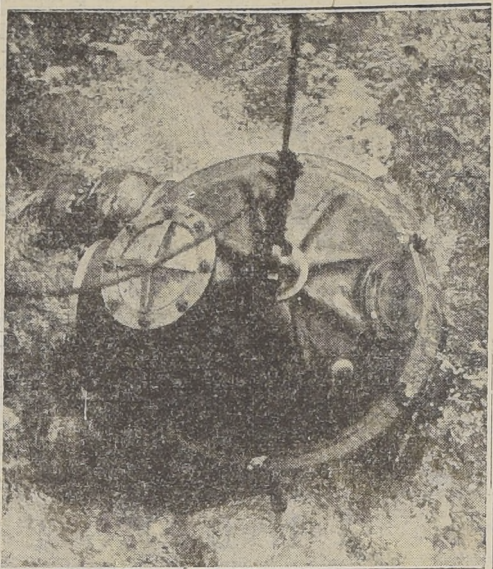
El robot de electrón, que costó 17,000 dólares, destinado a resistir la enorme presión submarina a 100 brazas de profundidad, desaparece por la borda del "Orphir". Dentro de él va el buzo Jim Jarrod. En la parte superior, puede verse una ventana de vidrio que permite el buzo mirar hacia arriba. También cuenta con idénticos medios de visión submarina a los costados y al frente del casco. A la derecha puede verse la parte superior de los tanques de oxígeno acoplados a la espalda del traje.
