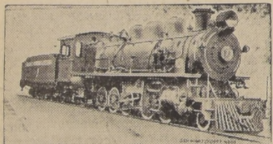
Locomotora de 3 cilindros y 100 mm. de via, construida para el F. C. de Iquique a Píntados
