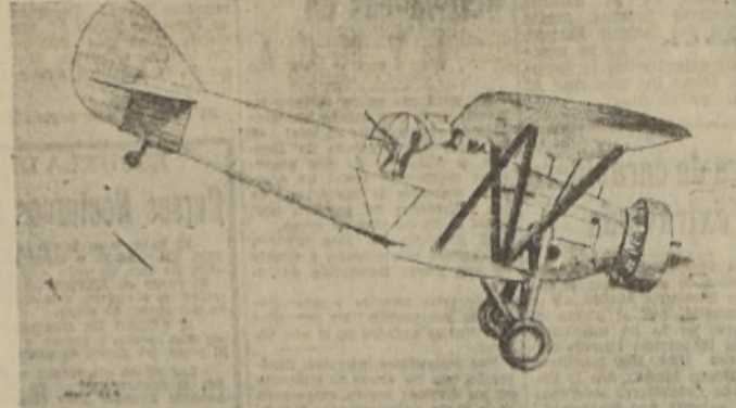
Fig. 4. "Bristol 120", un avión inglés para usos variados con moderno esqueleto de acero. Este aparato puede ser usado igualmente como biplaz de caza, bombardero ligero diurno, para exploración y foto-avión como también para amonaciones. La torre de ametralladora en forma de jaula, detrás del sitio del piloto, se llama "Parrot-cage" (jaula de papagayo).
