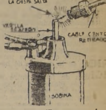
Método sencillo para probar la bobina de ignición
