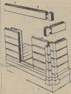
Esquema de montaje de la construcción en madera llamada maciza, en tabloncitos de 10x20.
