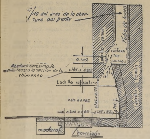
Sección de la chimenea
