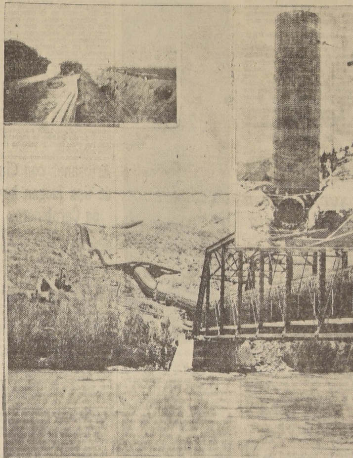
Una cañería de madera, de 6 pulgadas de diámetro, que muestra su gran adaptabilidad a los terrenos más irregulares. En el ángulo izquierdo: instalación de una cañería de madera, que funcionará bajo tierra. En el ángulo derecho: un estanque de gran capacidad, construido por el mismo sistema de dueñas de madera, utilizable también como silo, y que resulta mucho más barato, por cierto, que los silos de concreto.
