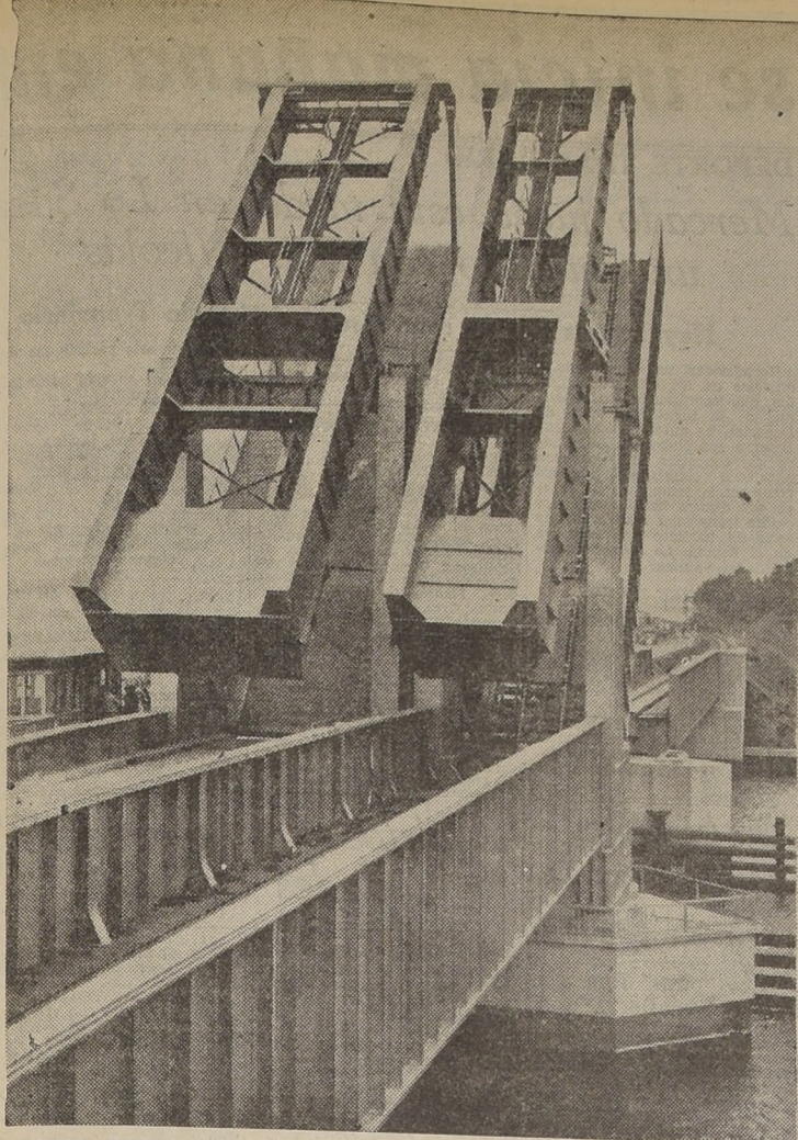
EL PUENTE BASCULANTE DEL DIQUE DE RUGEN, QUE PERMITE EL PASO DE GRANDES BUQUES
