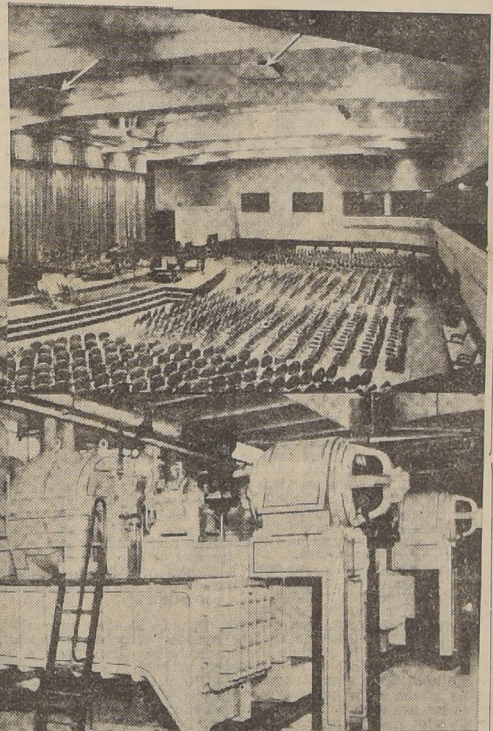
Una de las plantas de acondicionamiento del sistema "Carrier". Esta instalación supervisada por un experto norteamericano, envía el aire acondicionado por los conductos de la sala de espectáculos, para ser distribuido por los fabricantes y por el Surtinno Carrasco A. Ingeniero y agente exclusivo de "Carrier" el Teatro Metro, desde mañana se coloca a la altura de los cómodos teatros del mundo.
