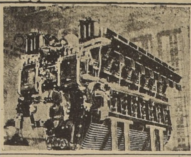
Este otro fué el de mayor tamaño y es uno de los que impulsarán al nuevo Zeppelin, actualmente en construcción
