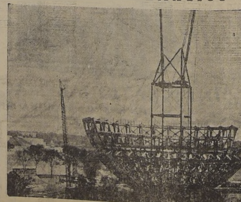
Una de las vigas en la construcción, a base de piezas metálicas corchadas. Periferia y el Trilón, monumento arquitectónico simbólico que forma el centro temático, motivo central de la grandiosa Feria
