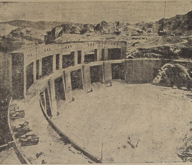
Una de las secciones, ya terminada, del gran dique Parker, que se construye en el río Colorado, 155 millas más abajo que el dique Boulder. Está destinada al control del agua necesaria para abastecer a la ciudad de Los Angeles y otras ciudades californianas.
