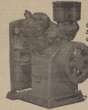
COMPRESORA SULLIVAN UNITAIR WL-60 REFRIGERADA POR AIRE
