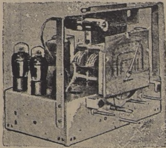
CHASSIS REFORZADO
