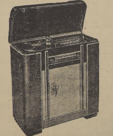
MODELO 862.— Radiogramófono de sobremesa. Circuito superheterodino de tres gamas de ondas. Equipo gramofónico de excepcional construcción con pick-up de gran sensibilidad.
