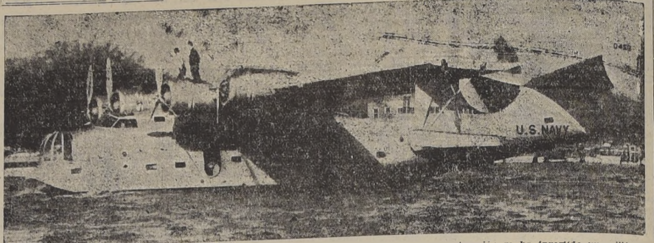
Gigantesco hidrovion experimental de bombardeo para la marina de costa, en cuya construcción se ha invertido un millón de dólares. Aparece en el canal de Washington, momentos antes de iniciar vuelo hacia San Diego. Tiene una envergadura de 115 pies, un largo de 77 y 28 de altura.
