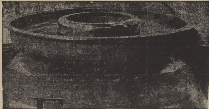
Paño para preparación de dinamita, prensada de una sola plancha de 19 mm. por la Lukens Steel Company (E. U.), para la E. I. de Pont de Nemours Co. (E. U.) Peso, 1360 kilos; diámetro, 3,25 metros.
