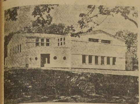
El curioso tipo de construcción, en cuya estructura se utilizaron arcos elásticos de madera laminada, colocados en secciones listas para emplearse.
