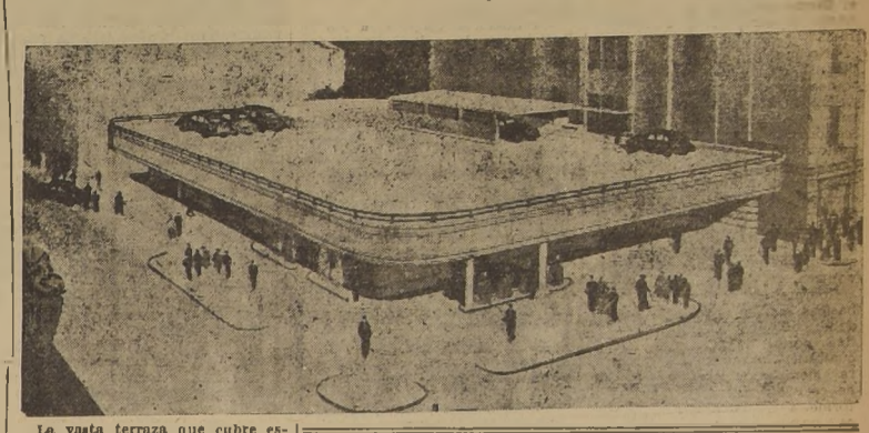
La vasta terraza que cubre esta nueva y original construcción, situada en el sector central de Nueva York y destinada a servir de estación de servicio para automóviles, ha sido dispuesta con el objeto de hacer posible el estacionamiento de un gran número de estos vehículos, los que suben a ella por medio de una rampa helicoidal, cuya entrada se encuentra en el primer piso.
