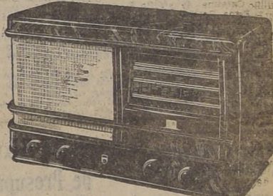
MODELO 635 V.—Superheterodino "Reflex" de batería, con válvulas de red y de funcionamiento perfecto. Opera por medio de un acumulador de 6 Volt, combinado con un silento especial Philips. Conmutador economizador de corriente, que permite reducir el consumo normal de la batería en un 50% al escuchar las estaciones potentes.
