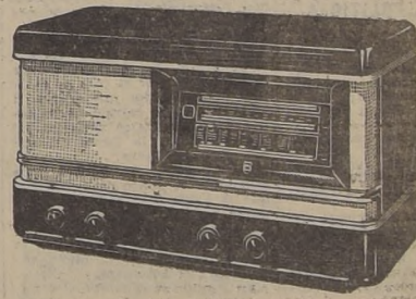
MODELO 314.—Superheterodino equipado con corrección automática de calidad. Nuevo circuito de contrarreactión para la pureza del tono. Condensador de sintonización termostático. Sobrio gabinete de madera, con adornos de metal.
