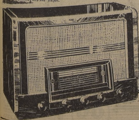
Modelo 316: Superheterodino de bajo consumo con sintonización de bandspread calibrado. Sintonizador de permeabilidad y dial calibrado en bandas de 13, 15, 20, 25 y 30 metros. Amplificación especial de los bajos.
