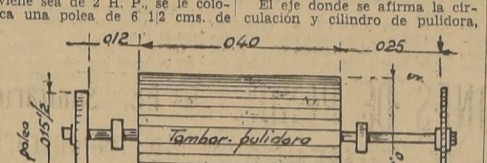
Figura 2. puede ser un palier viejo de automóvil. Tendrá 2 rodamientos, los que asientan en los huecos que se practican en los tirantes del armazón de la mesa; en un extremo se coloca la polea de 155 cms. de diámetro y, en el otro, la sierra circular. El tambor para la pulidora se hará de madera y colocará 2 discos; a la vez, se puede hacerle al eje una perforación, a fin de pasar un pasador, para que dichos discos no patinen, y
