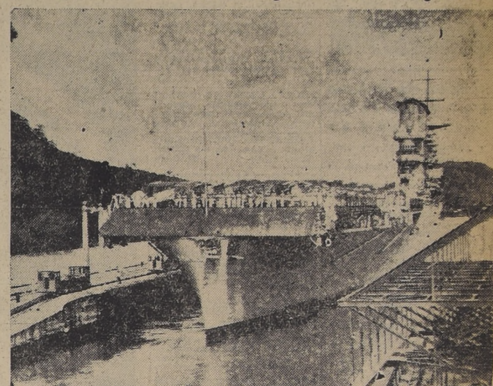
El portaaviones "Saratoga" cruzando las esclusas de Pedro Miguel (Canal de Panamá). Este gran portaaviones, gemelo del "Lexington", desplaza 33,000 toneladas y tiene capacidad para transportar 79 aviones de combate. Su armamento principal consiste en 8 cañones de 8 pulgadas, y 12 de 5, además de numerosas piezas antiaéreas. Su andar es de 33.91 nudos por hora.
