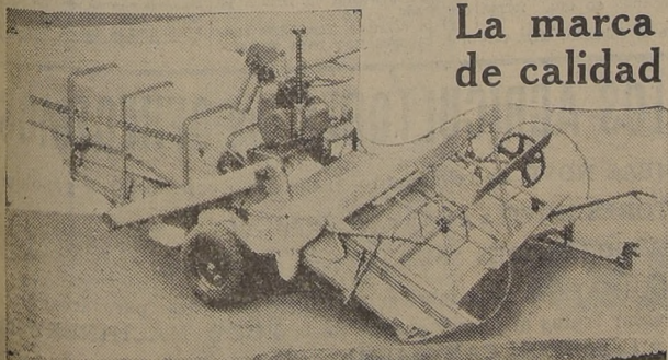
COSECHADORA "CASE" MODELO A-6
