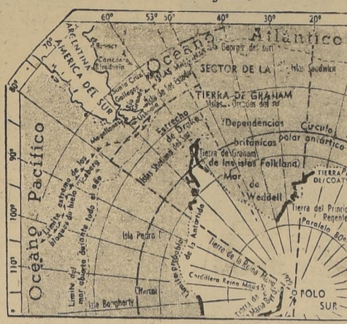
En este esquema cartográfico se puede apreciar el ángulo formado por los meridianos 53 y 90 grados oeste de Greenwich.
