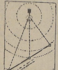
El diseño muestra cómo distribuye el ejército sus puestos de observación sísmica para localizar una batería enemiga. Se determinan las direcciones que convergen hacia el lugar donde se originan las ondas sísmicas, y se conocen las distancias y ángulos de las bases. El resto, como puede deducirse, es simple geometría.
