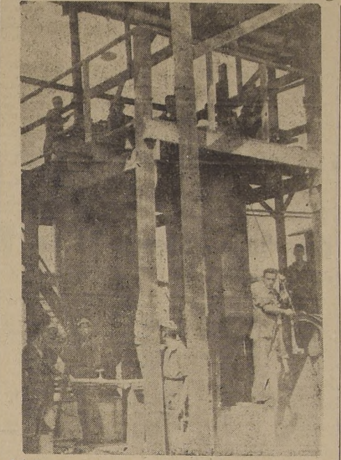
Autoclaves en que se sigue el proceso de recuperación de las materias grasas
